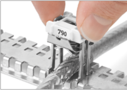
Montaż obejmy zaciskowej do ekranu ze sprężyną na perforowanej szynie montażowej TS 35 ① ② ③ ④ ⑤ ⑥ ⑦ ⑧ ⑨ ⑩ ⑪ ⑫ ⑬ ⑭ ⑮ ⑯ ⑰ ⑱ ⑲ ⑳
