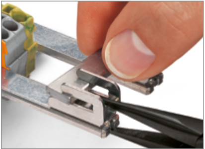
W celu demontażu szyny zbiorczej należy ścisnąć obcęgami sprężynę dociskającą szynę ④ ⑤ ⑥ ⑦ ⑪ ⑫ ⑬ ⑭ ⑮ ⑯ ⑰ ⑱ ⑲ ⑳
