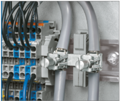
Obejmy zaciskowe do ekranu na szynie równoległej do szyny montażowej z przewodzącą stopką na TS 35 ④ ⑤ ⑥ ⑦ ⑪ ⑫ ⑬ ⑭ ⑮ ⑯ ⑰ ⑱ ⑲ ⑳
