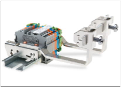
Szyna zbiorcza usytuowana pionowo mocowana na metalowym wsporniku do przesuwanego uchwyty teowego ④ ⑤ ⑥ ⑦ ⑪ ⑫ ⑬ ⑭ ⑮ ⑯ ⑰ ⑱ ⑲ ⑳
