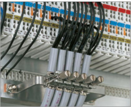
Obejmy zaciskowe do ekranu ze śrubą na wyprofilowanej miedzianej szynie zbiorczej ④ ⑤ ⑥ ⑦ ⑪ ⑫ ⑬ ⑭ ⑮ ⑯ ⑰ ⑱ ⑲ ⑳
