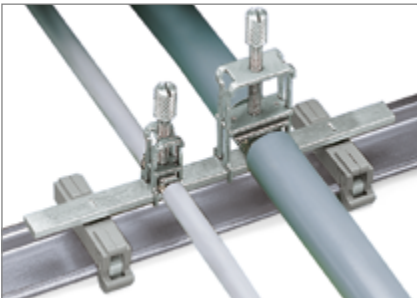
Obejmy zaciskowe do ekranu ze śrubą na szynie równoległej do szyny montażowej z 2 przewodzącymi stopkami na TS 35 ④ ⑤ ⑥ ⑦ ⑪ ⑫ ⑬ ⑭ ⑮ ⑯ ⑰ ⑱ ⑲ ⑳
