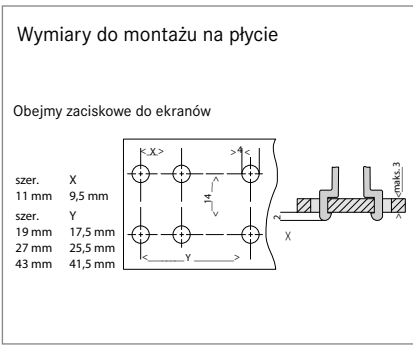
Wymiary [mm] ④ ⑤ ⑥ ⑦
