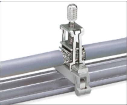
Obejma zaciskowa do ekranu ze śrubą na szynie prostopadłej do szyny montażowej z przewodzącą stopką na TS 35 ④ ⑤ ⑥ ⑦ ⑪ ⑫ ⑬ ⑭ ⑮ ⑯ ⑰ ⑱ ⑲ ⑳
