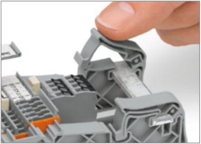
Montaż szyny zbiorczej na izolowanych wspornikach ④ ⑤ ⑥ ⑦ ⑪ ⑫ ⑬ ⑭ ⑮ ⑯ ⑰ ⑱ ⑲ ⑳
