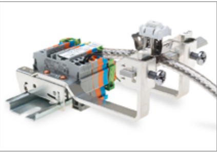
Obejma zaciskowa do ekranu ze sprężyną na szynie zbiorczej usytuowanej poziomo mocowanej na metalowym wsporniku do przesuwanego uchwyty teowego ① ② ③ ④ ⑤ ⑥ ⑦ ⑪ ⑫ ⑬ ⑭ ⑮ ⑯ ⑰ ⑱ ⑲ ⑳
